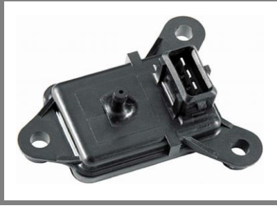
Hava Basınç Sensörü Sensor, Intake Manifold Pressure (MAP) SLX-PALIO
